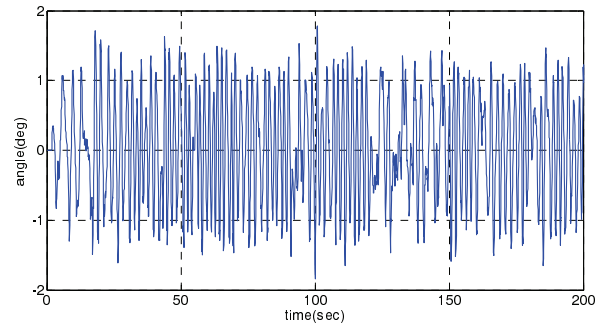
그림 4. 전형적인 DOB에서 롤 각.
