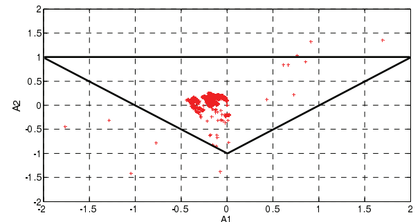
그림 9. 역 공칭모델 안정성.
